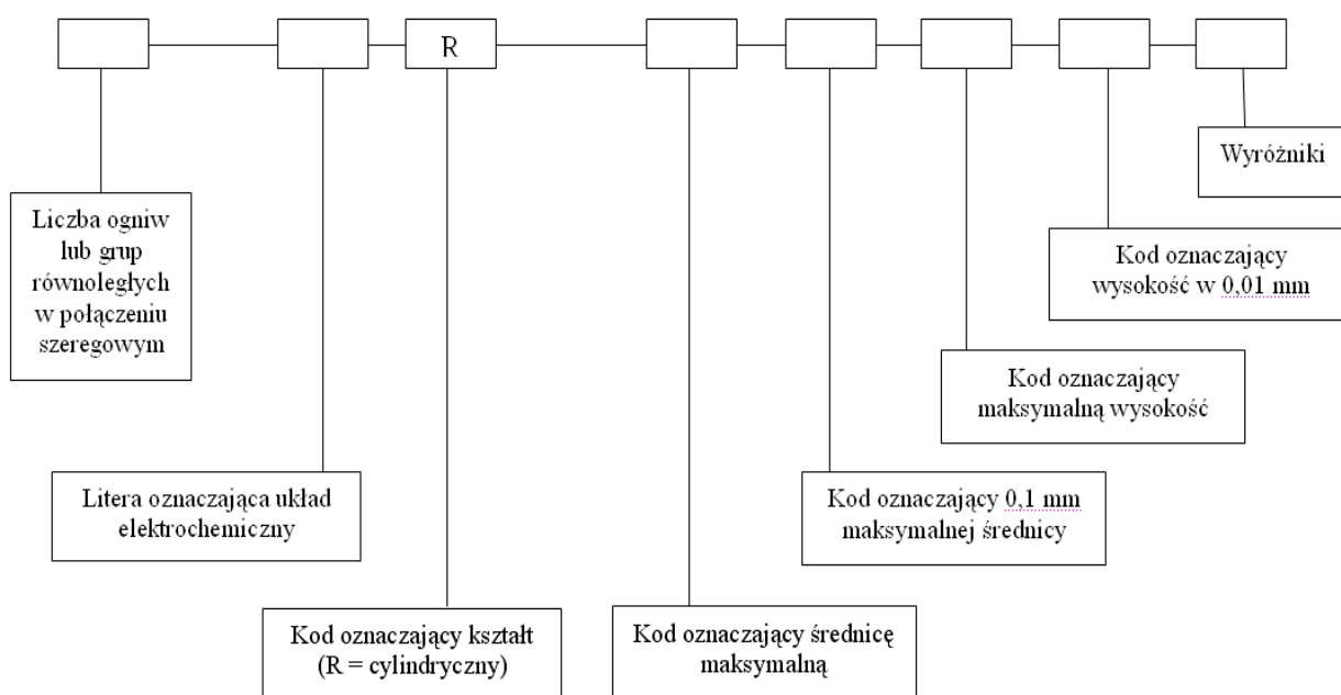
Schemat 1. Baterie cylindryczne o średnicy i wysokości mniejszej od 100 mm
